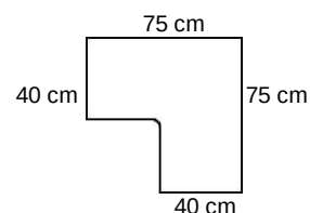
Draufsicht - Eckteil
